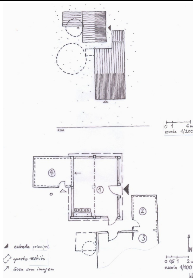
8.3. Planta baixa
