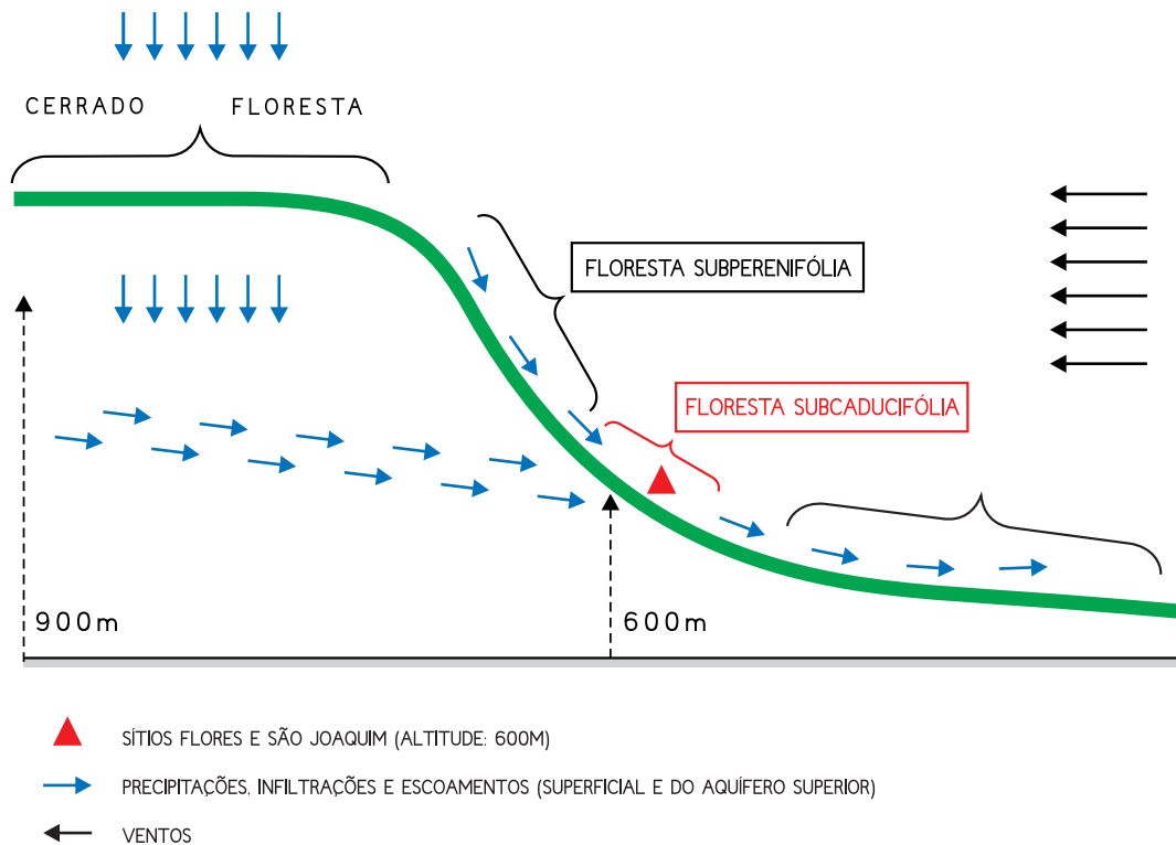
GRÁFICO 1 PERFIL GEOMORFOLÓGICO DA BACIA SEDIMENTAR DO ARARIPE E FATORES QUE CONDICIONAM O DESENVOLVIMENTO BIOLÓGICO DAS ÁRVORES (SILVA & CARDOSO, 2011)
